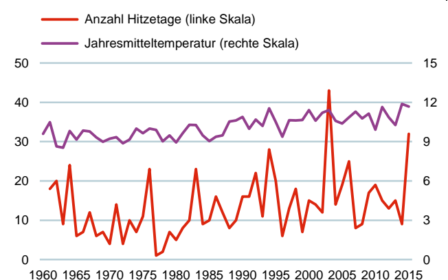
Abb.6-12; Quelle: Meteorologischer Verein der Region Basel; Bundesamt für Meteorologie und Klimatologie MeteoSchweiz.
